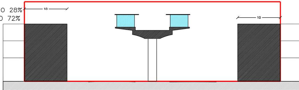
SECCION TIPO METRO ELEVADO AV. PRIMERO DE MAYO ENTRE AV. 68 Y NQS ESTACIÓN ROSARIO
