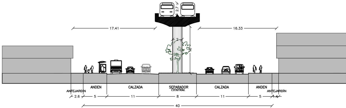
SECCION TIPO METRO ELEVADO AV. PRIMERO DE MAYO
