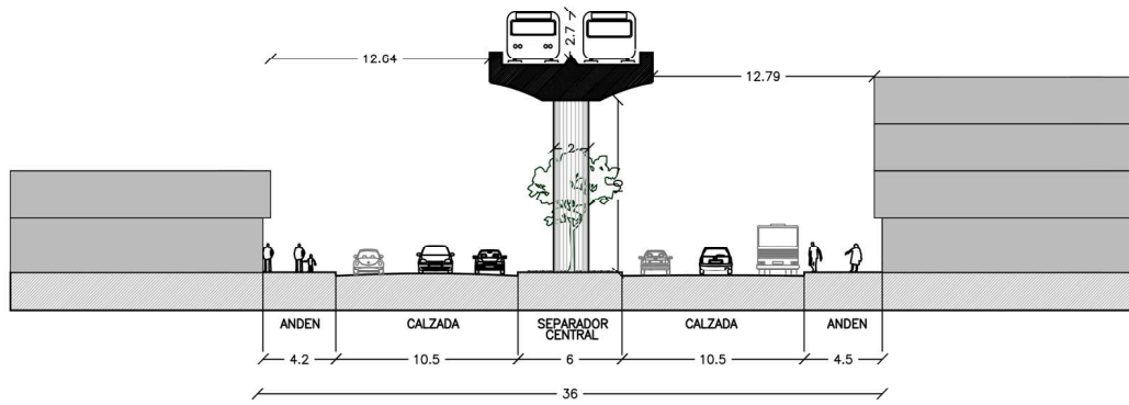
SECCION TIPO METRO ELEVADO AV. VILLAVICENCIO
