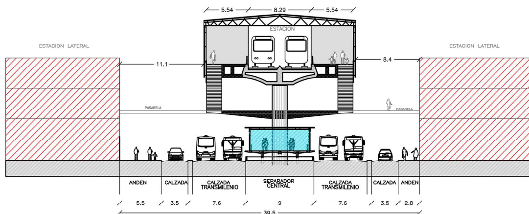
CARACAS— ESTACIÓN CALLE 57— CASO ESTRECHO
