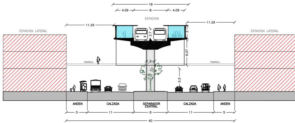
SECCION TIPO METRO ELEVADO AV. PRIMERO DE MAYO ENTRE AV. 68 Y NQS ESTACIÓN ROSARIO
