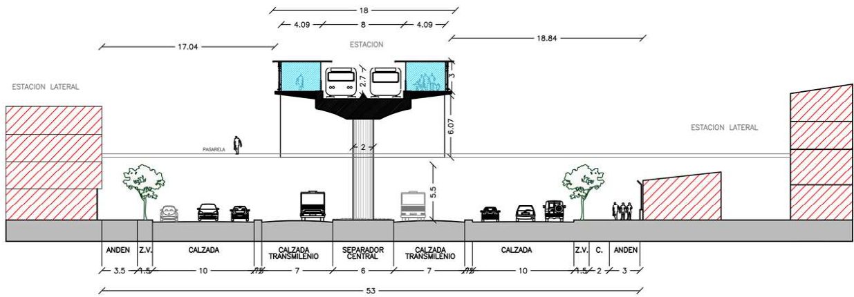
SECCION TIPO METRO ELEVADO AUTOSUR ENTRE AV. 1ro DE MAYO Y CALLE 8 SUR ESTACIÓN NQS
