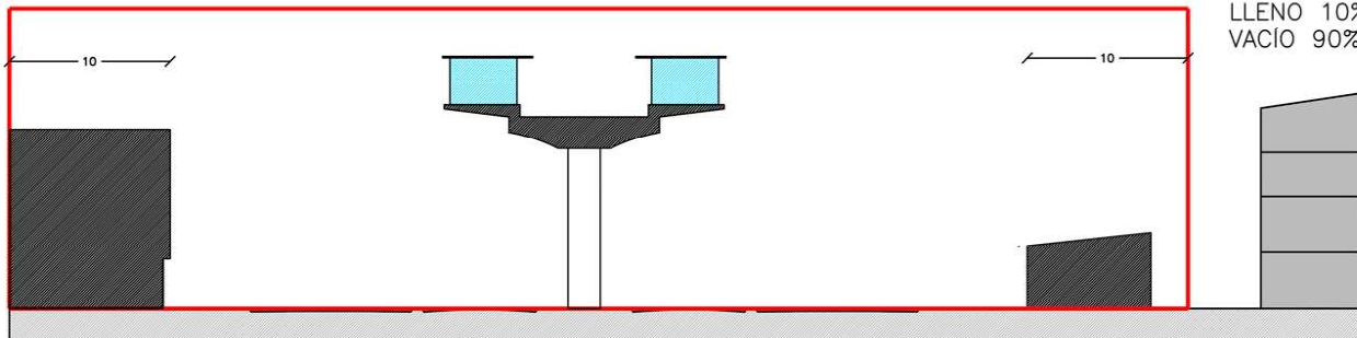
SECCION TIPO METRO ELEVADO AUTOSUR ENTRE AV. 1ro DE MAYO Y CALLE 8 SUR ESTACIÓN NQS
