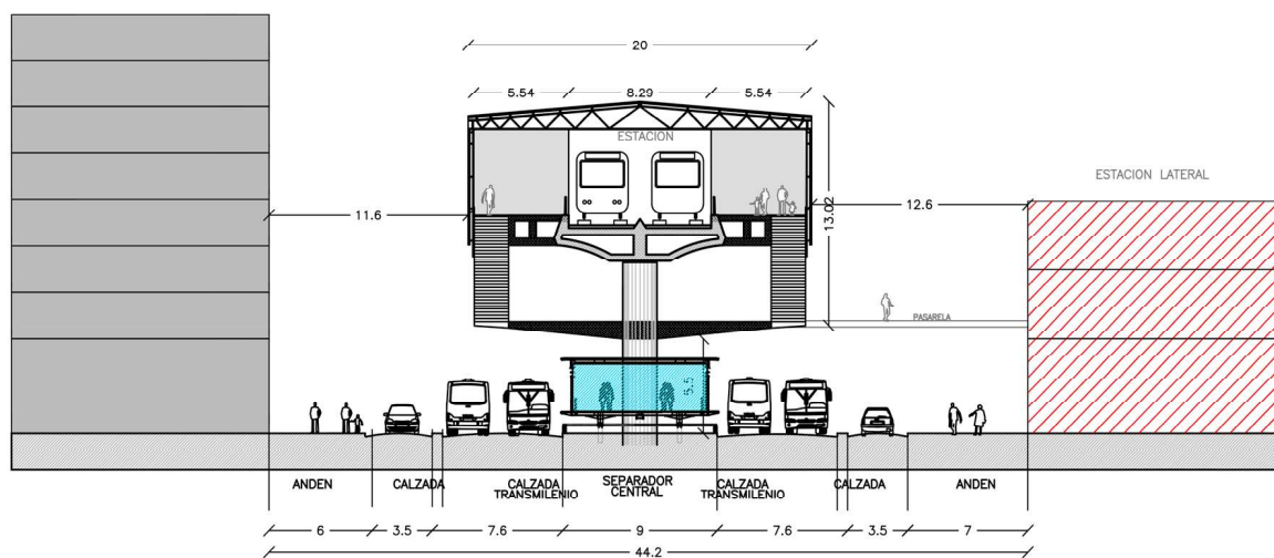
CARACAS— ESTACIÓN CALLE 57— CASO AMPLIO
