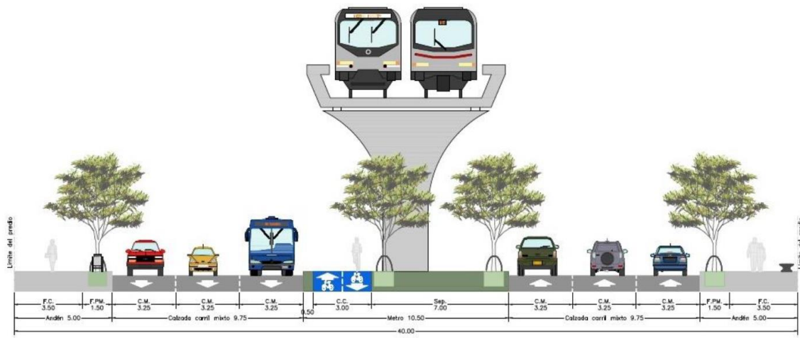
Figura 7.82 Sección transversal en la Avenida Primera de Mayo entre la Avenida Ciudad de Villavicencio y la Avenida Norte Quito Sur (NQS)
