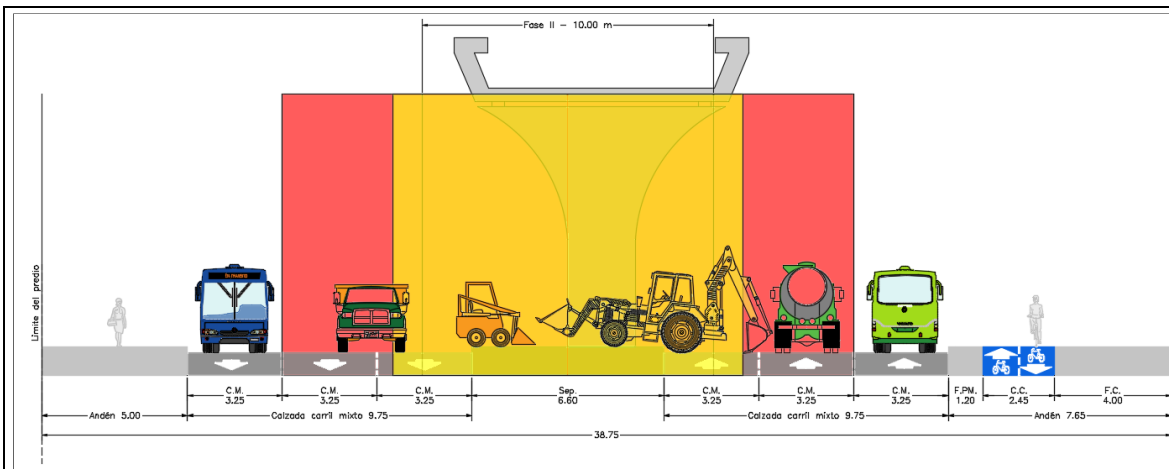
Figura 7.68 Sección transversal típica con afectación en Fase II
