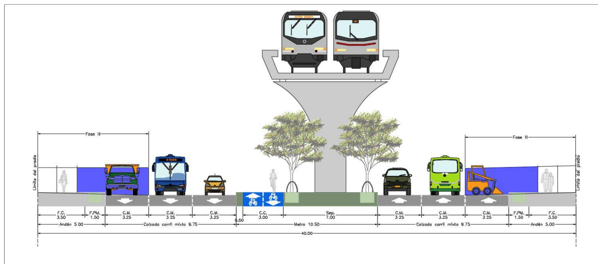
Figura 7.69 Sección transversal típica con afectación en Fase III
