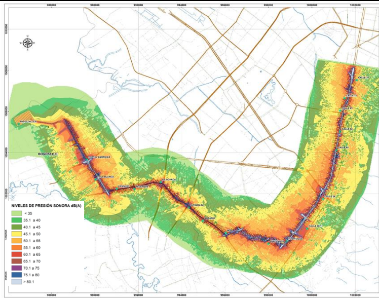
Figura 7.50 Isófona nocturna escenario construcción proyecto-línea base
