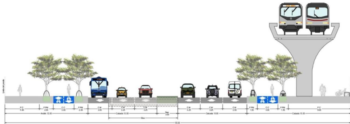
Figura 7.81 Sección transversal en Avenida Ciudad de Villavicencio entre la futura Avenida Longitudinal de Occidente y la Avenida Ciudad de Cali.
