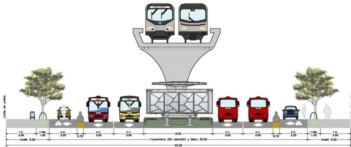
Figura 7.83 Sección transversal a nivel de estación en la Avenida Caracas entre la Calle 26 y la Calle 76 Fuente: Con base en Lineamientos de Espacio público para la Estructuración Técnica del Tramo 1 de la Primera Línea de Metro de Bogotá
