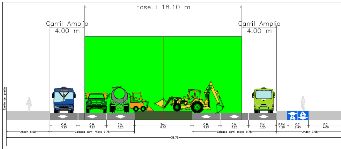
Figura 7.67 Sección transversal típica con afectación en Fase I
