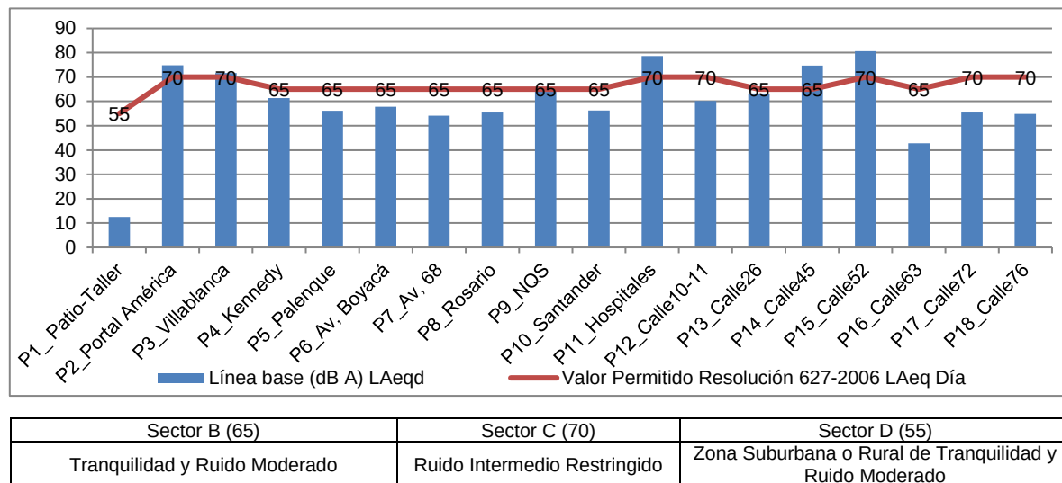
Figura 7.95 Niveles de ruido ambiental horario diurno
