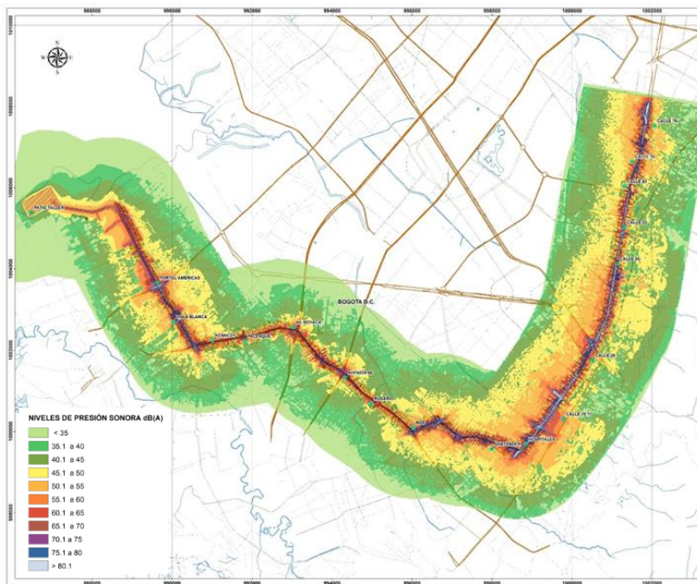
Figura 7.49 Isófona diurna escenario construcción proyecto-línea base
